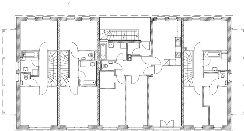
1. Obergeschoss, Haus A
