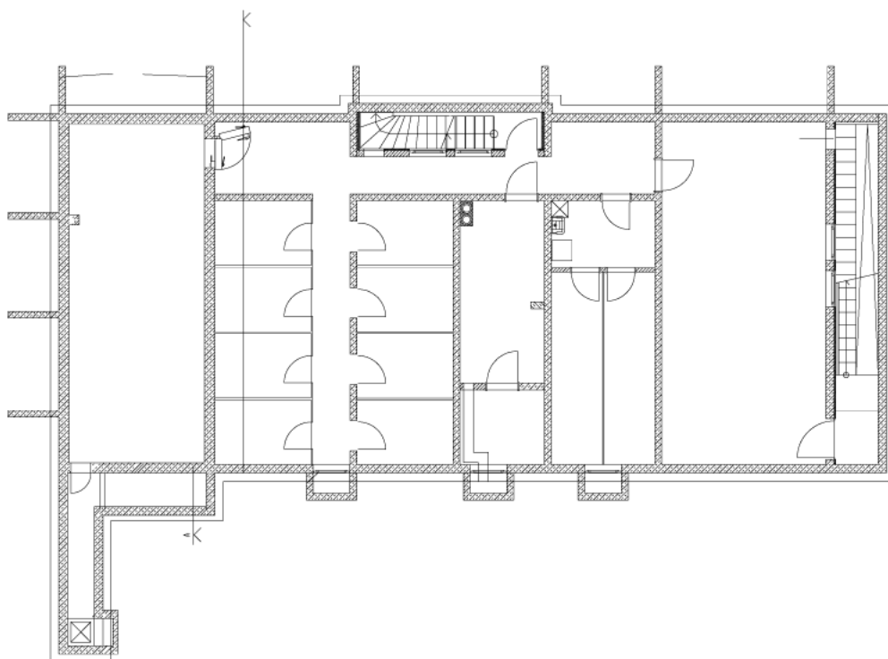
1. Obergeschoss, Haus A
