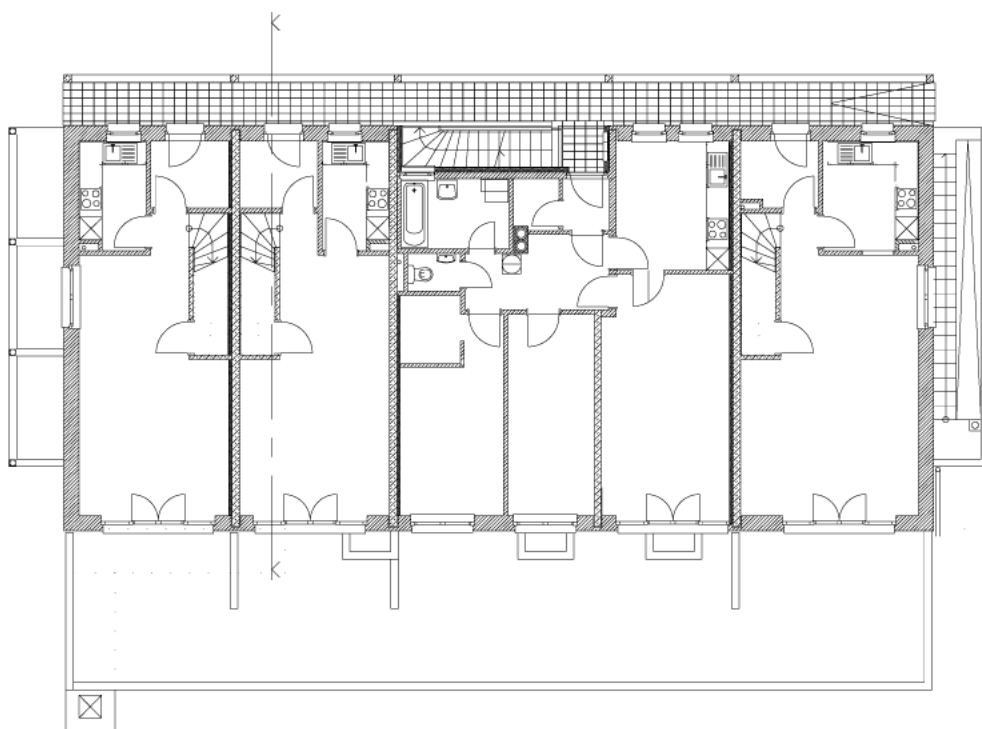
Erdgeschoss, Haus A
