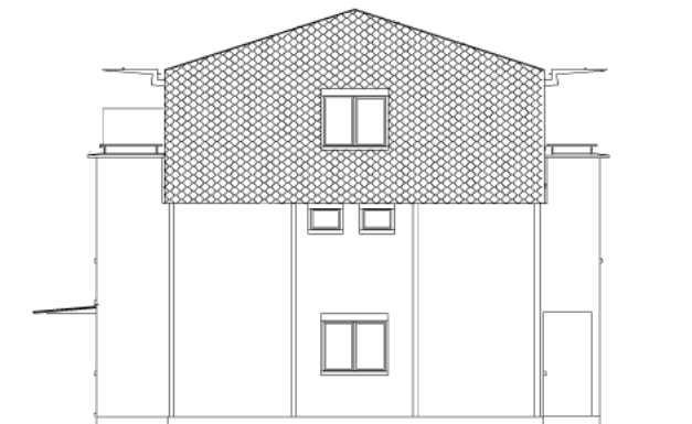
Ansicht Ost
