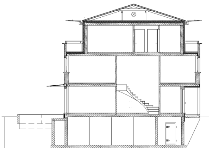
Schnitt A-A, Haus A
